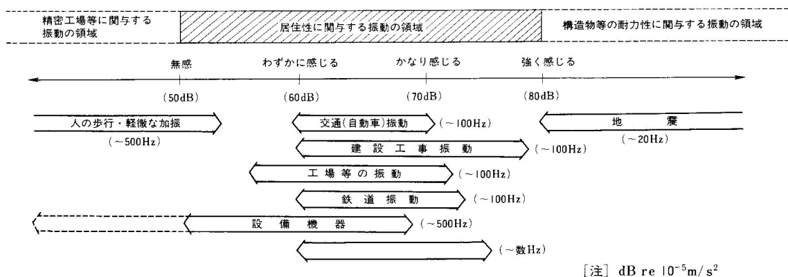
図 環境振動の種類と範囲（出典：参考文献4）
