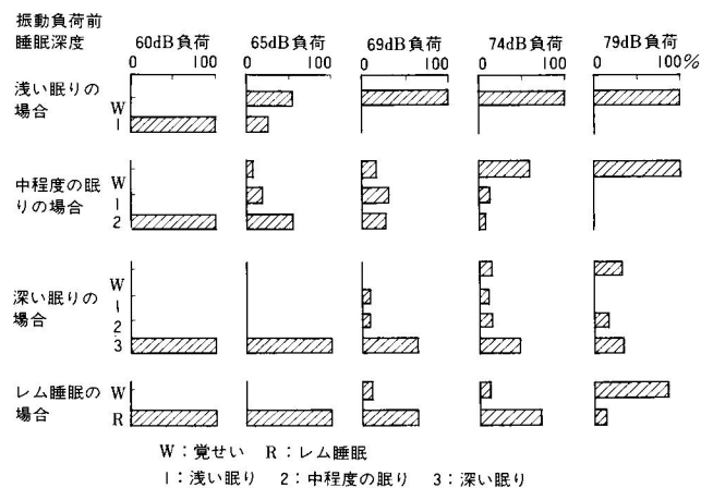
図 振動の睡眠に及ぼす影響（列車振動を前提としたもの）（出典：参考文献4）
