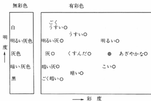
図 無彩色の明度ならびに有彩色の明度および彩度の相互関係 (JIS Z 8102-1985)
