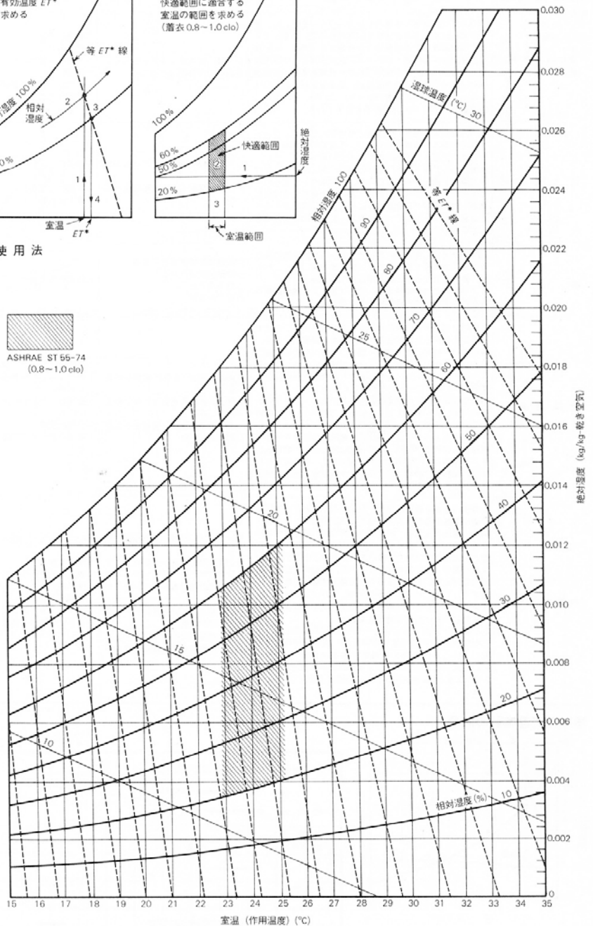
快適線図と新有効温度 ET^* (ASHRAE)*1 [1]
